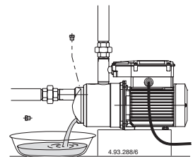
Fig. 5 Scarico Draining Entleerung Vidange Vaciado Vuttapping Aftappen Αποστράγγιση Слив 排空
