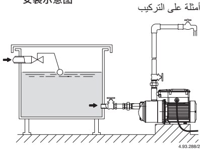
Fig. 1 Funzionamento sotto battente Positive suction head operation Zulaufbetrieb Fonctionnement en charge Funcionamiento bajo carga Tillrinning sugsidan Toeloopsituatie
